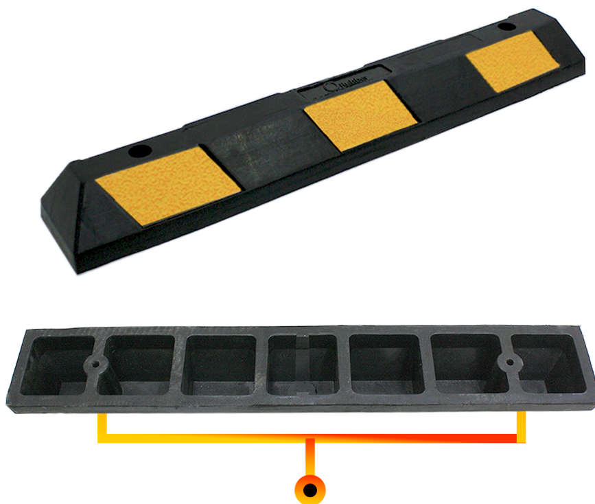
ORIFICIOS INSTALACIÓN
